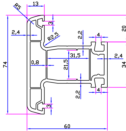
60 MULLION SERİE
